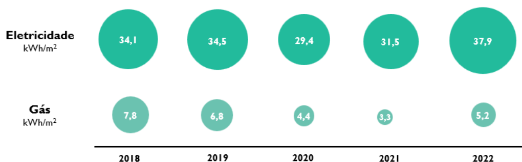
Figura 5: consumos de energia por área utilizada
